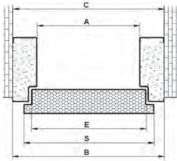
Ościeżnica drzwi
