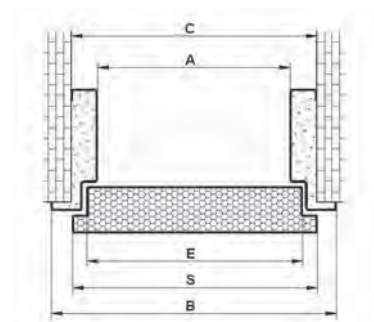
Ościeżnica drzwi
