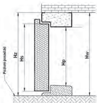
Ościeznica drzwi, próg
