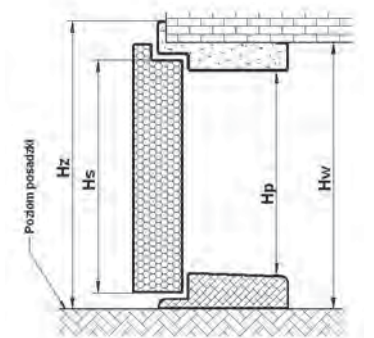
Ościeżnica drzwi, próg
