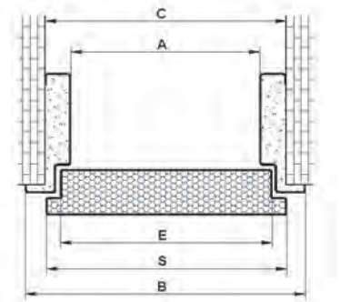
Ościeżnica drzwi
