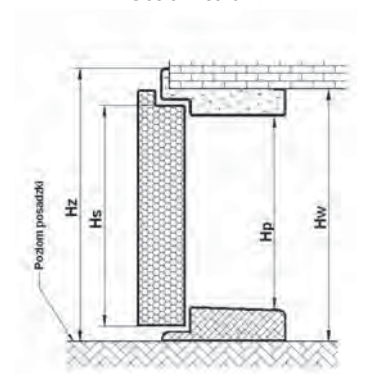
Ościeżnica drzwi, próg
