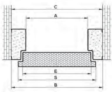
Ościeżnica drzwi
