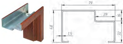
OŚCIEŻNICA ASYMETRYCZNA BEZ USZCZELKI FB (do drzwi TT i GTT)
