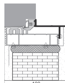
SARA PLUS M z aluminiowym elementem maskującym
