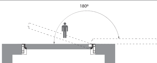
SARA G do ściany gipsowo-kartonowej
