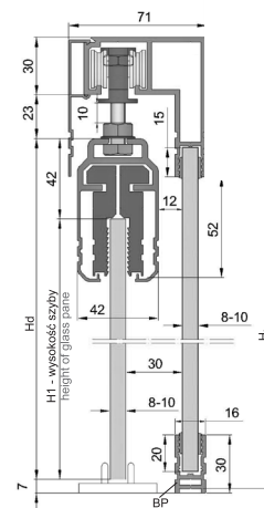
OPCJA: drzwi szklane mocowane w dużych szczękach UD
