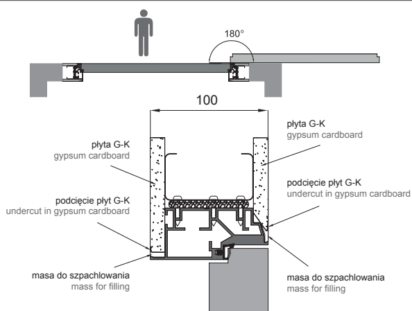
SARA EXTRA G do ściany gipsowo-kartonowej
