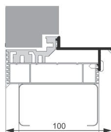
SARA PLUS M z aluminiowym elementem maskującym
