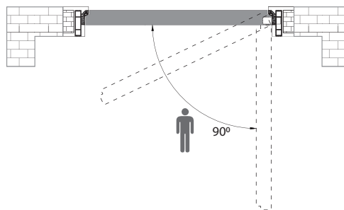
SARA PLUS M z aluminiowym elementem maskującym
