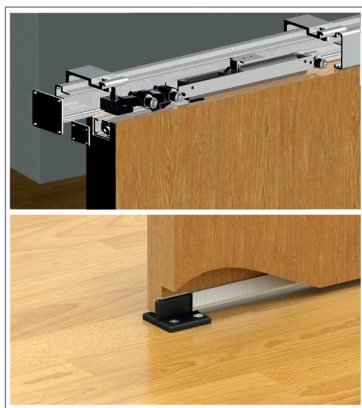
SPAZIO B do skrzydeł drewnianych
