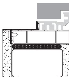
SARA PLUS M z aluminiowym elementem maskującym
