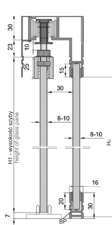
OPCJA: drzwi szklane mocowane w małych szczękach UM
