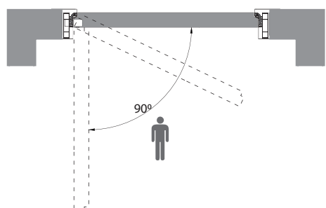
SARA PLUS M z aluminiowym elementem maskującym
