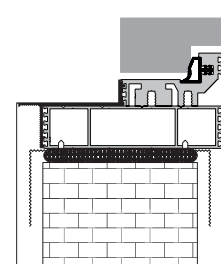
SARA PLUS M z aluminiowym elementem maskującym
