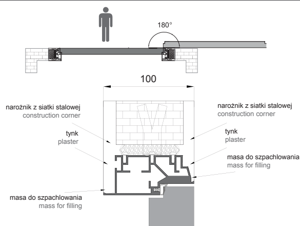
SARA EXTRA M do ściany murowanej
