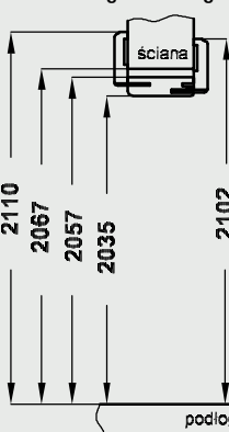
Przekrój pionowy tunelu regulowanego
